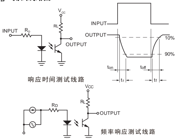
Fig.1 测试线路图
