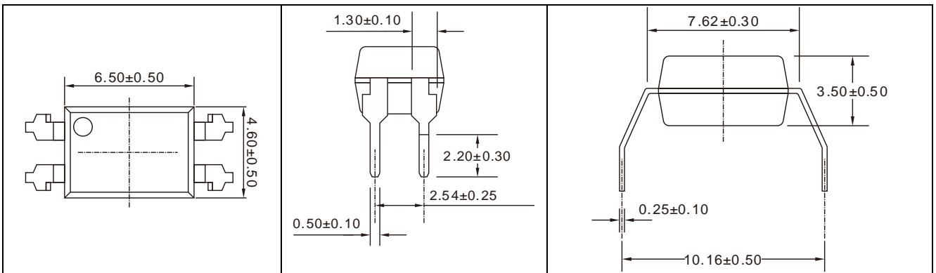
DIP-M-4
