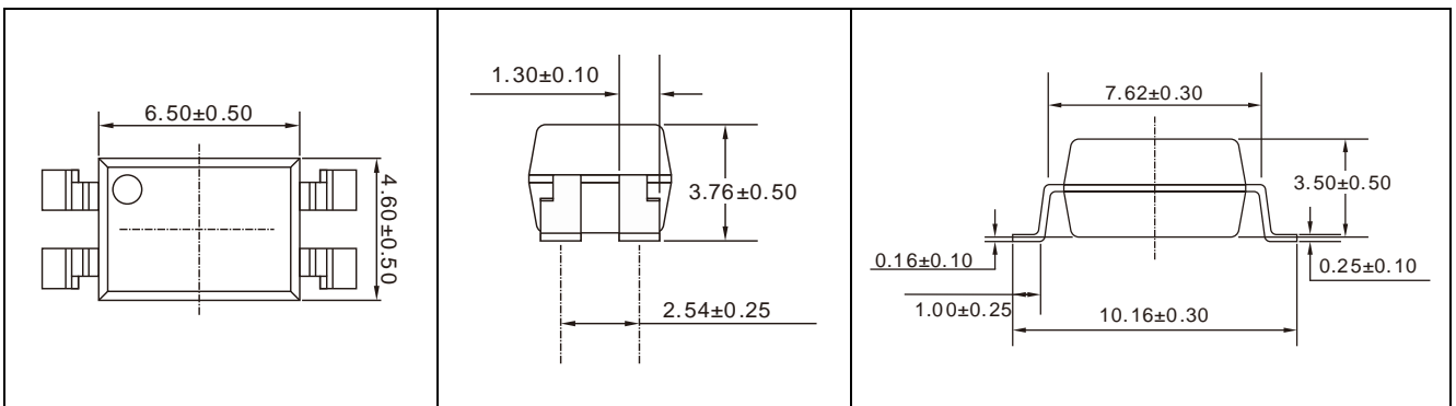
SMD-4
