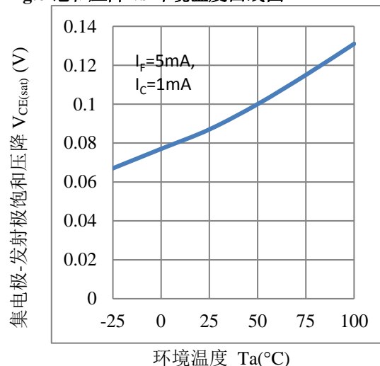
Fig.6 饱和压降 vs 环境温度曲线图
