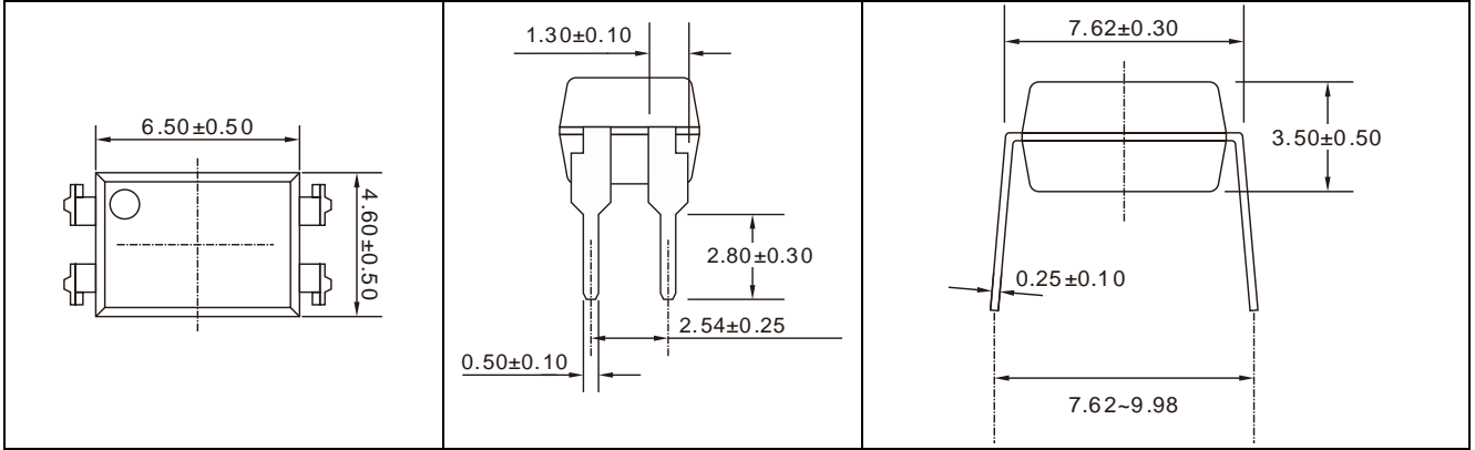
DIP-4
